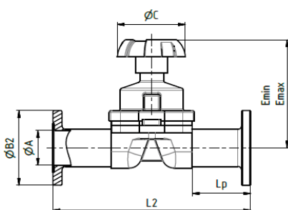
Мембранный клапан ПН-ПН Membránový ventil PN - PN
