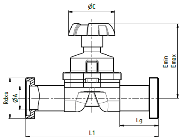
Мембранный клапан Г - Г Membránový ventil G - G
